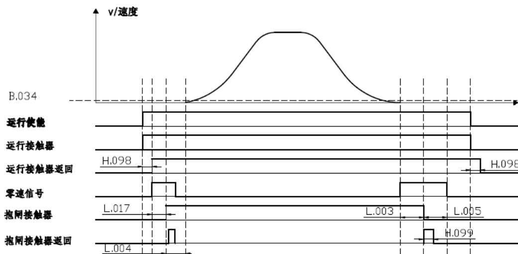
图 6-8 电梯正常运行时序图
