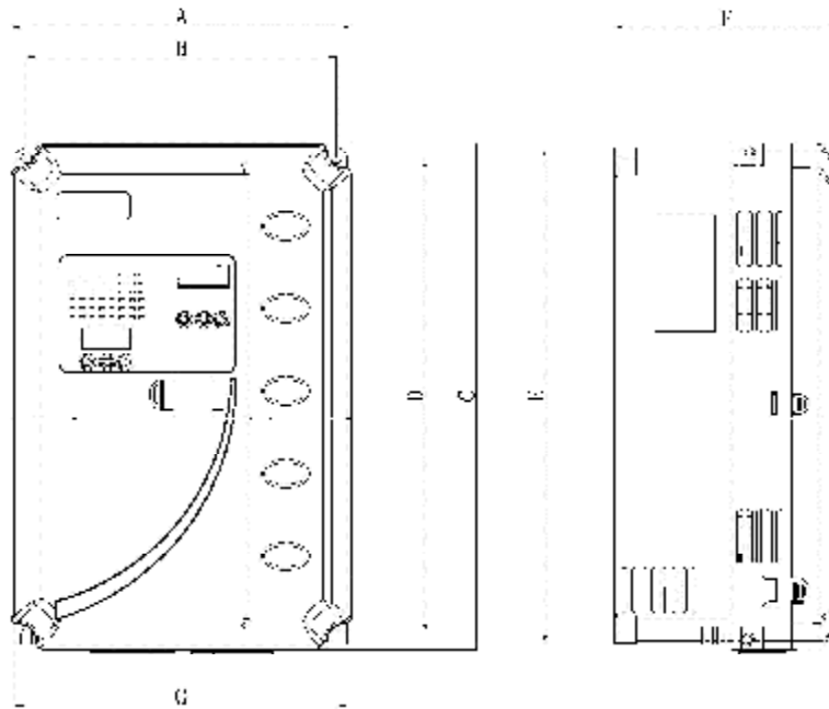
图 2-1 Size A~B 安装尺寸图
