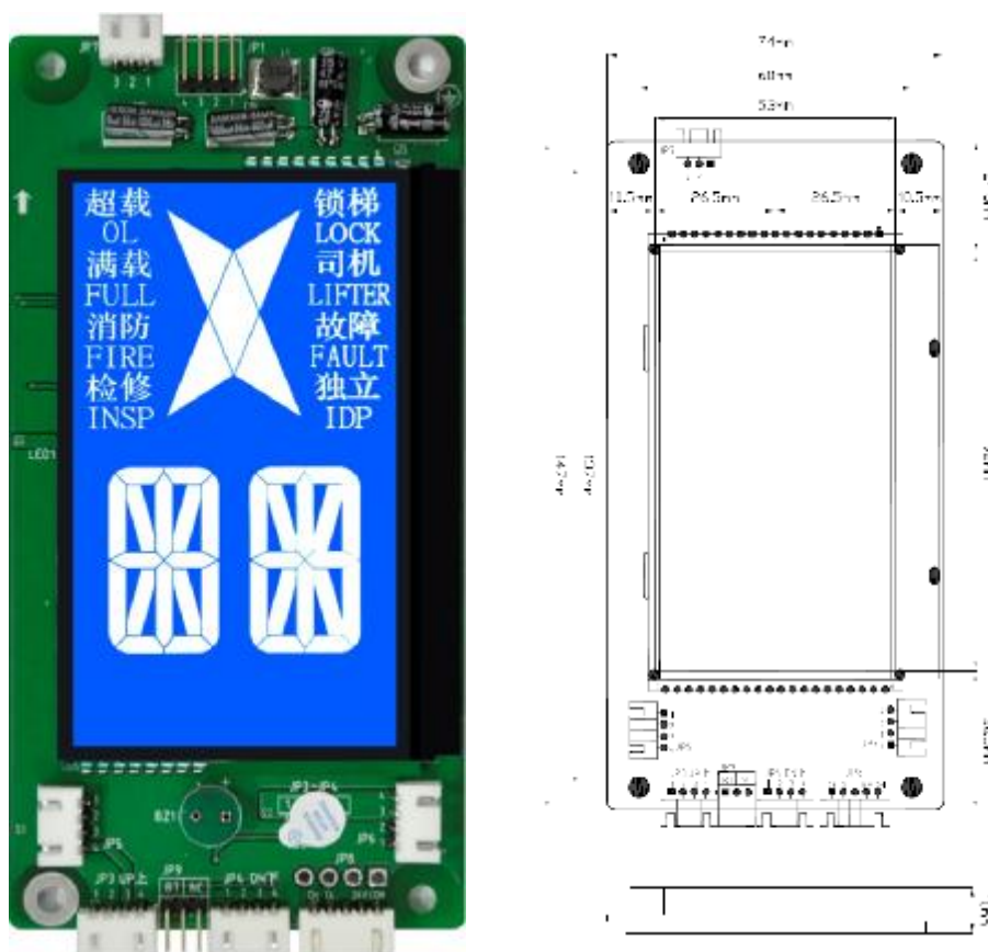
图 4.4.2.2.1 FHS0BW-0 外观及尺寸
