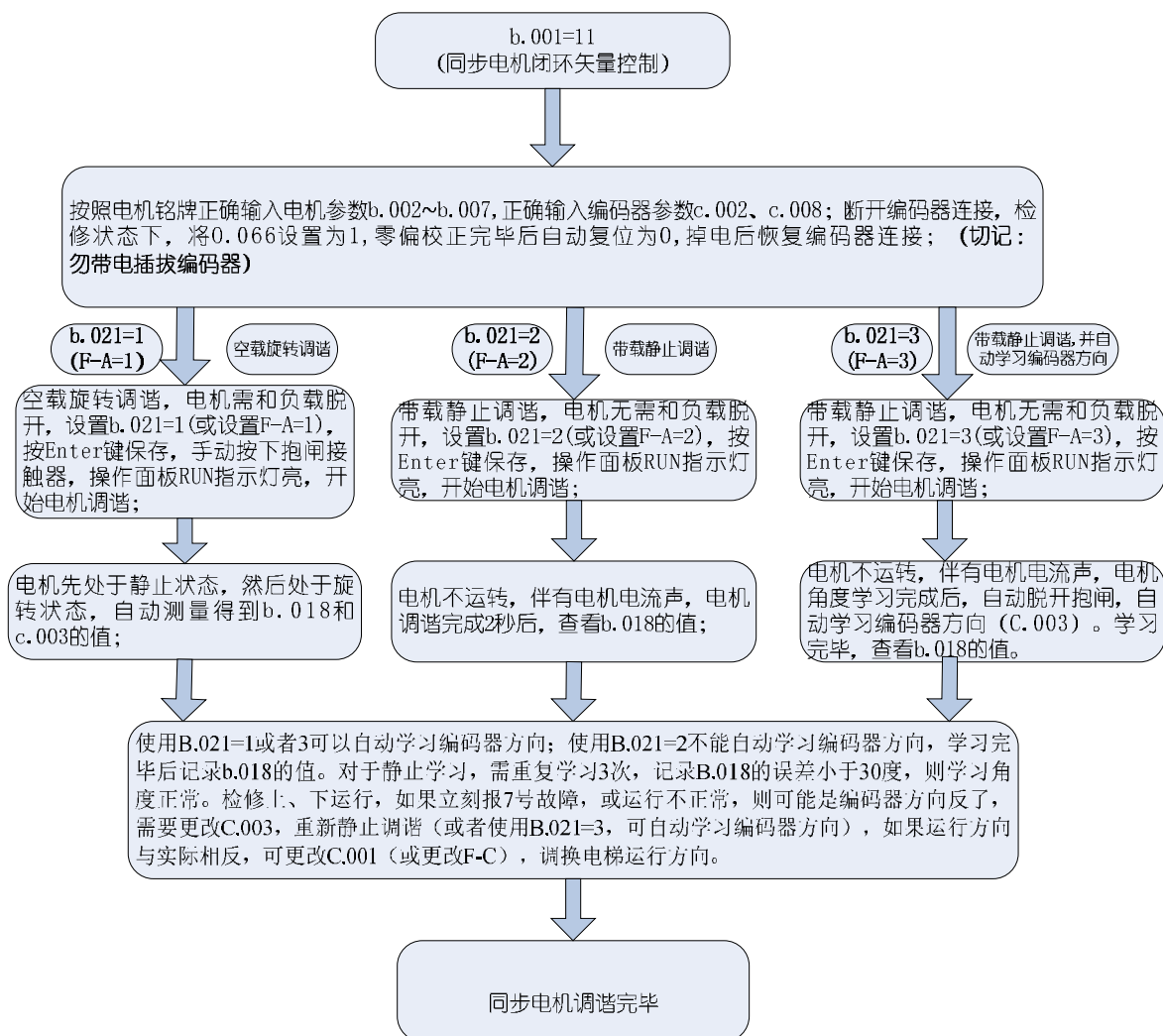
图 5-2-4-3 同步电机调谐简易流程
