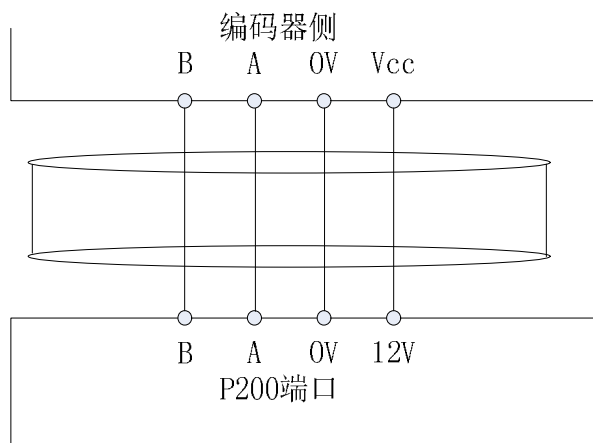
图 3-5-2-1 异步编码器卡接线方式
