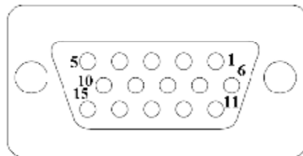
图 3-5-1 P500 DB15 各针脚顺序
