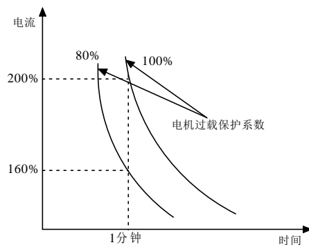
图 6-1 电机过载保护曲线图
