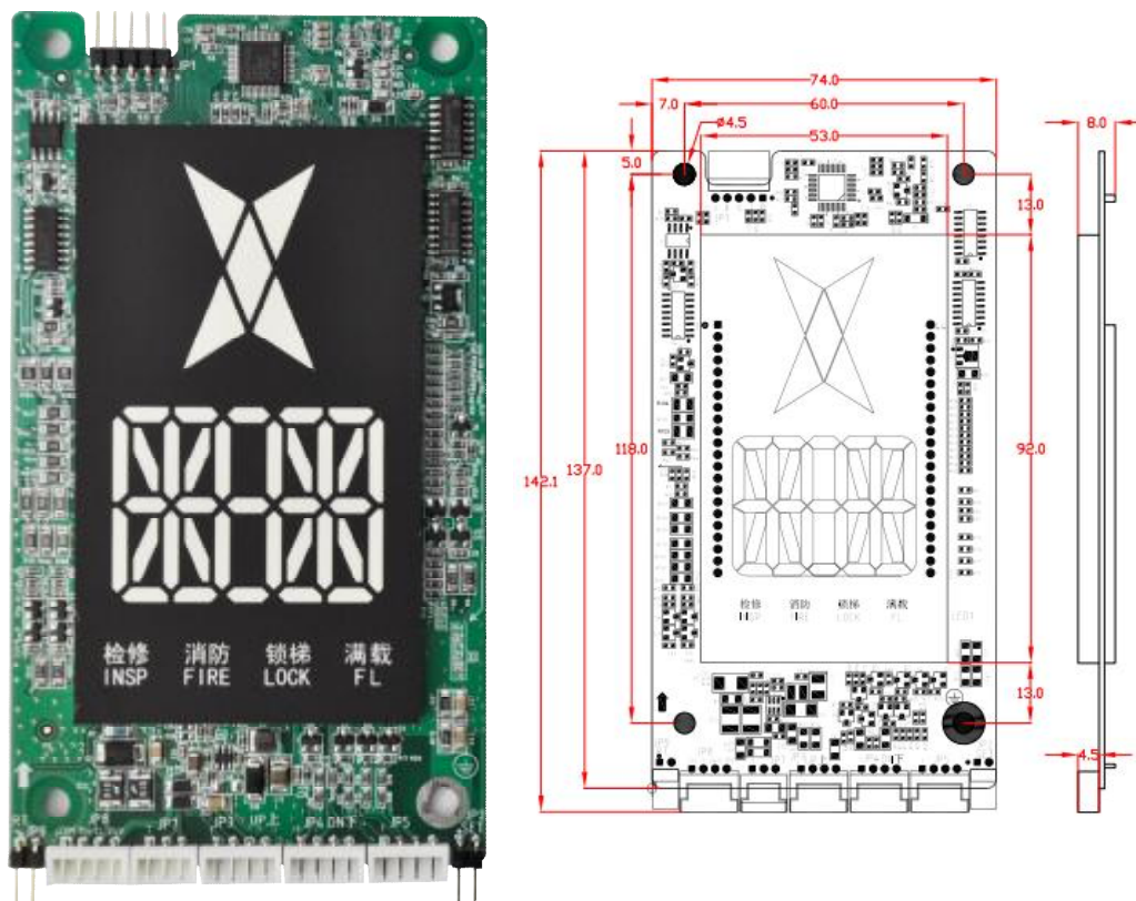
SW-HB-L1 外形尺寸
