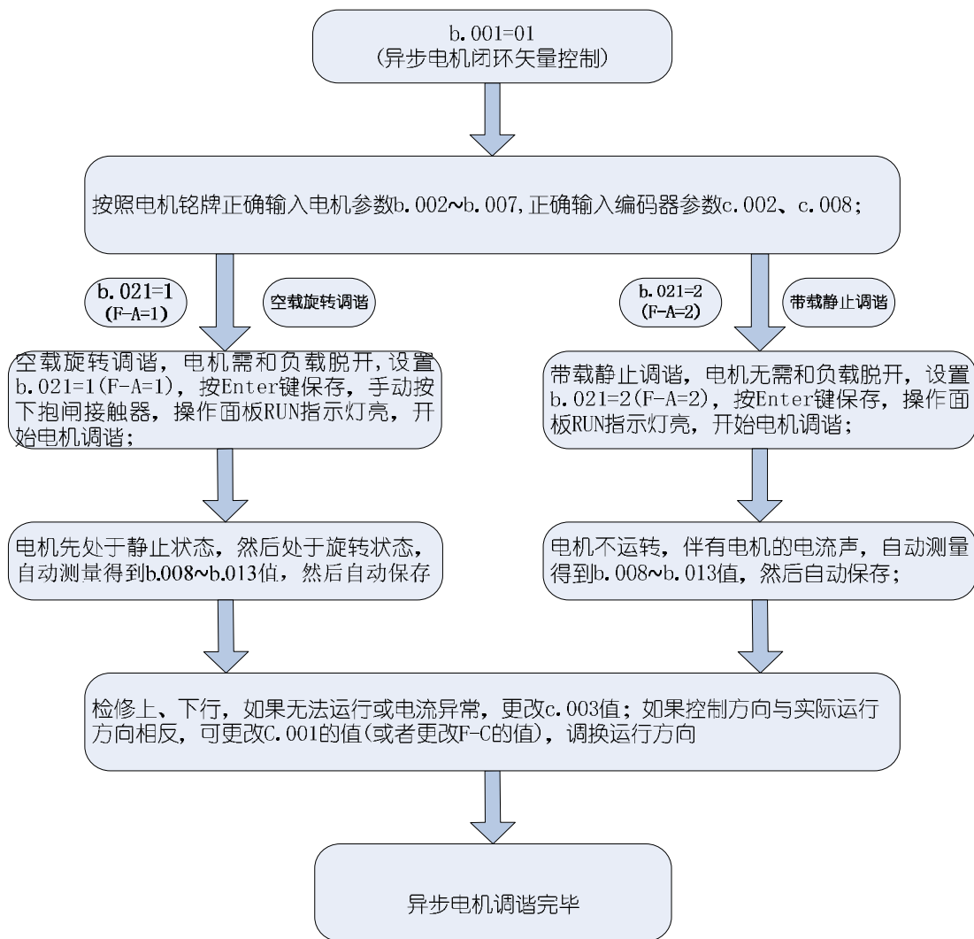
图 5-2-4-2 异步电机调谐简易流程
