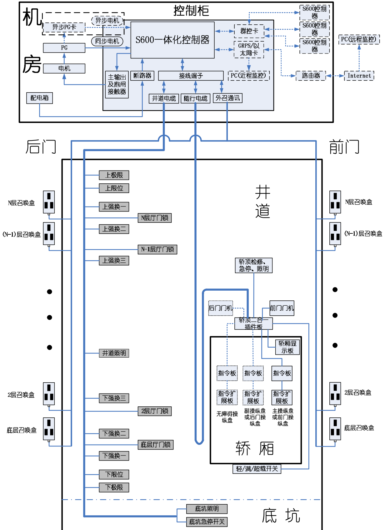
图 3-1 系统典型配置框图
