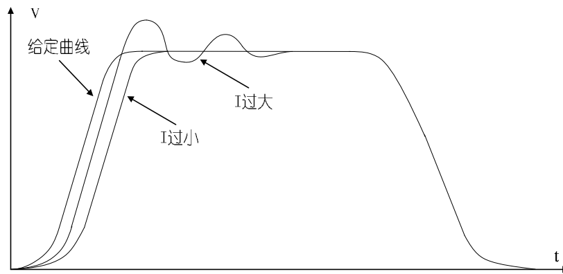
图 6-10 积分常数 I 对反馈跟踪的影响
