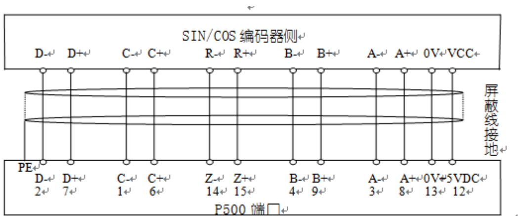
图 3-5-1.1 正余弦编码器配线图
