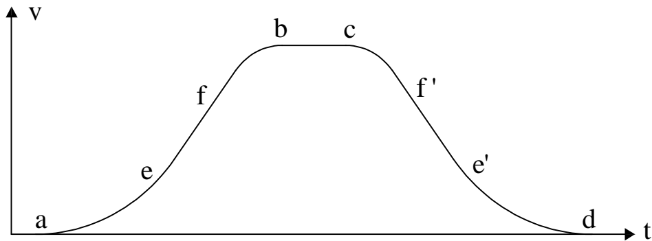
图 6-6 运行曲线分段示意图
