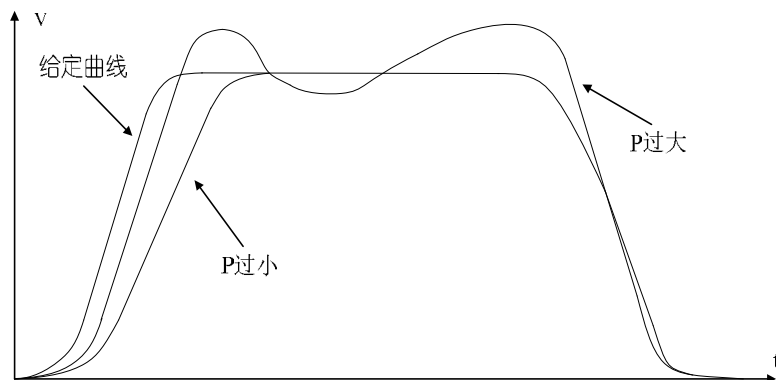
图 6-9 比例常数 P 对反馈跟踪的影响
