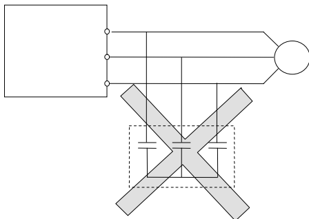
图 1-2 变频器输出端禁止使用电容器
