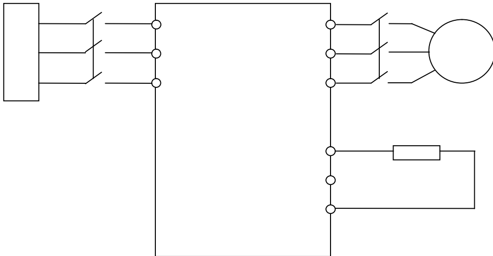
图 3-3-1 主回路接线图
