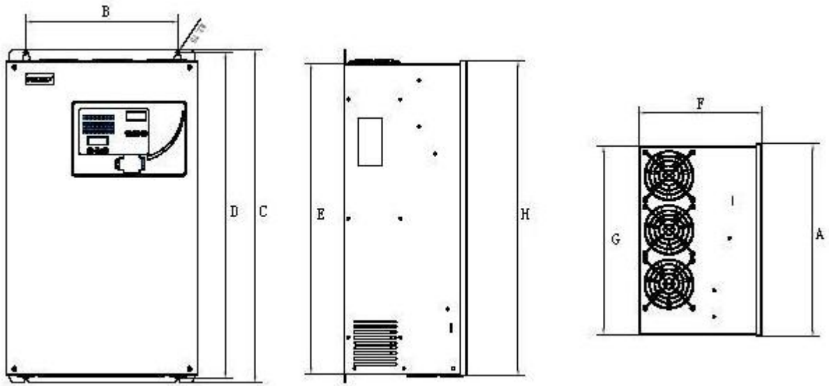
图 2-2 Size C 安装尺寸图
