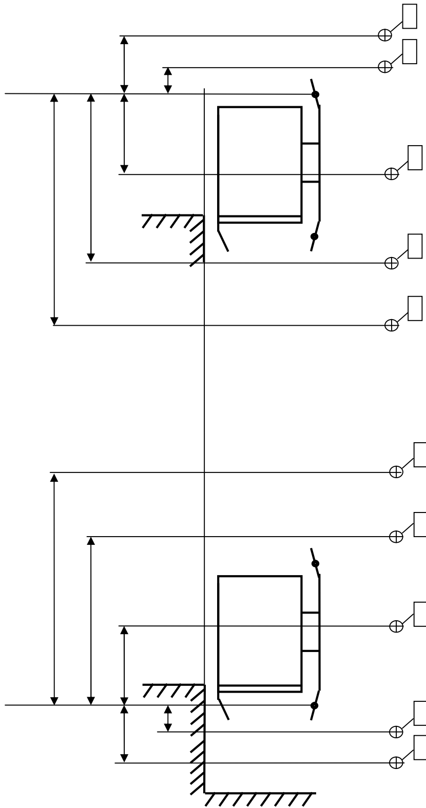
图3-2-2-2 井道强换开关安装位置
