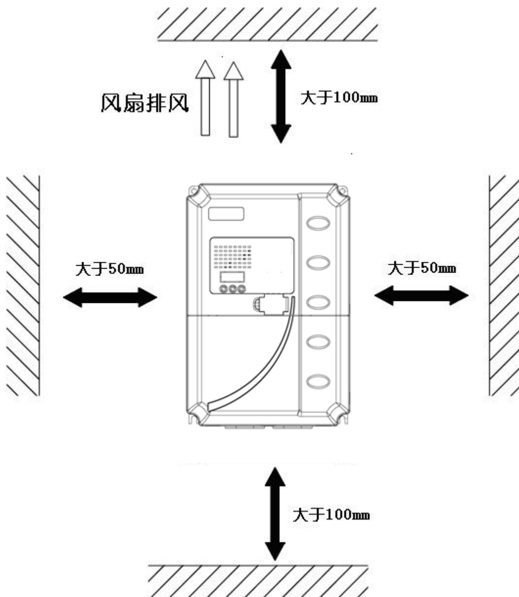
图 2-3 安装间隔距离(Size C 及以下)
