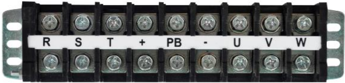
图 3-3-2 SIZE C 主回路端子排列
