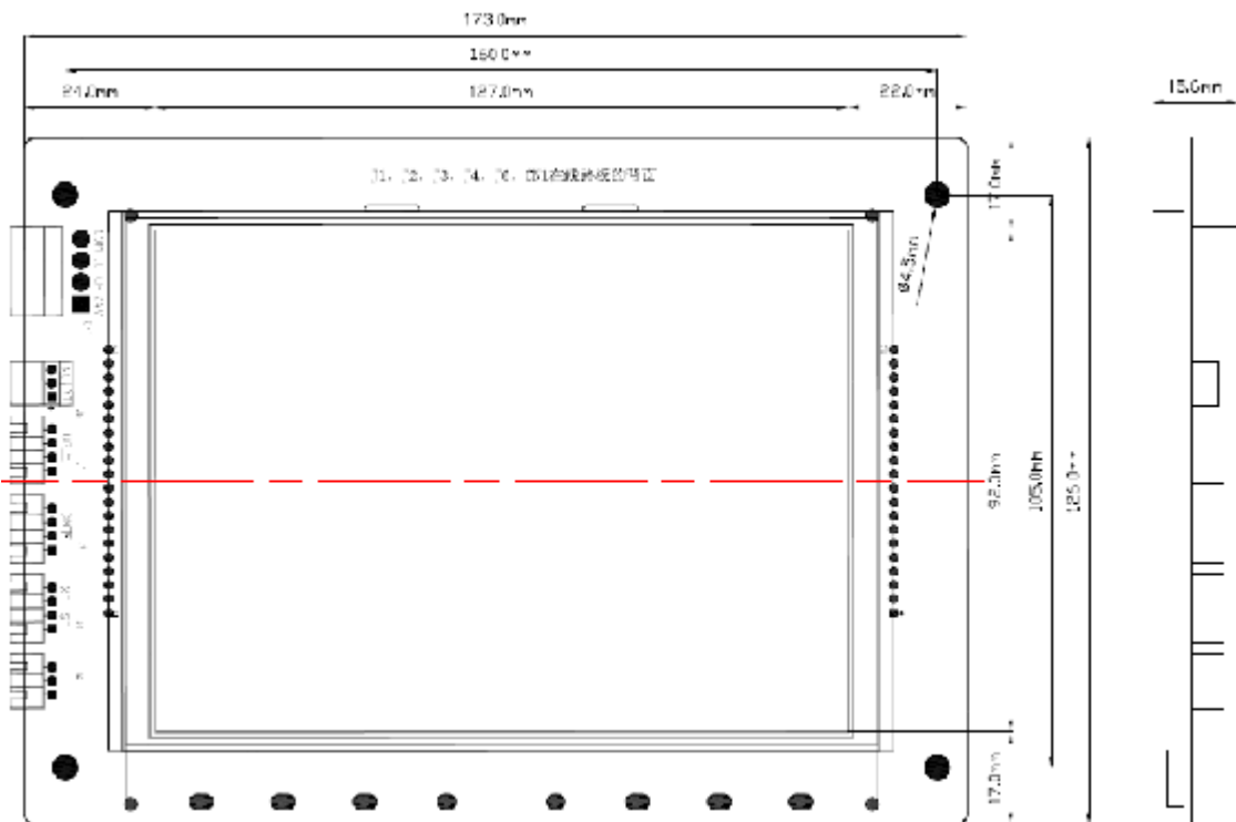
FHS1BW06-0 尺寸图
