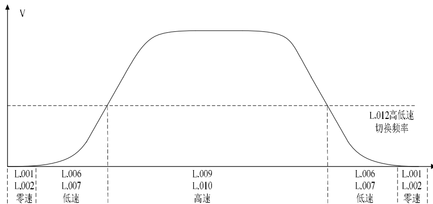
图 6-11 电梯运行曲线分段 PI 控制图
