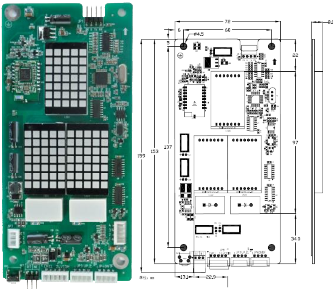
SW-HB-L00 外观及尺寸
