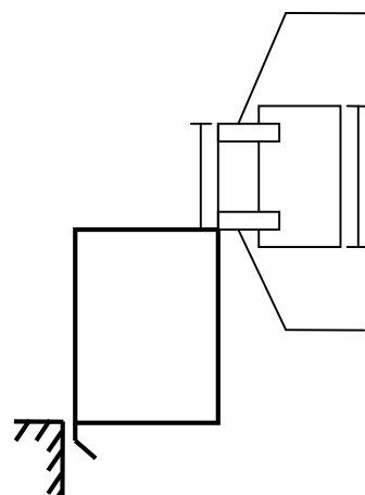
图3-4 安装2个平层开关
