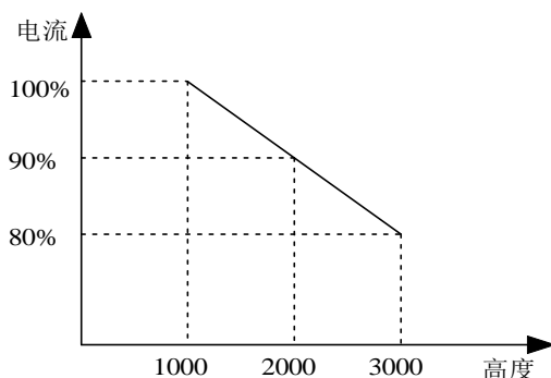
图 1-3 变频器额定输出电流与海拔高度降额使用
